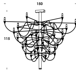
150/pl30 30 E14 max 10w
