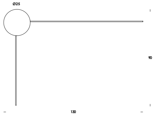
80-120/sp rettangolo aperto - diffusore Ø25 E27 max 60w
