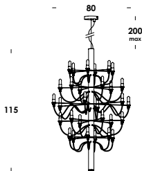
80/s30 30 E14 max 10w
