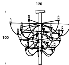
120/pl24 24 E14 max 10w
